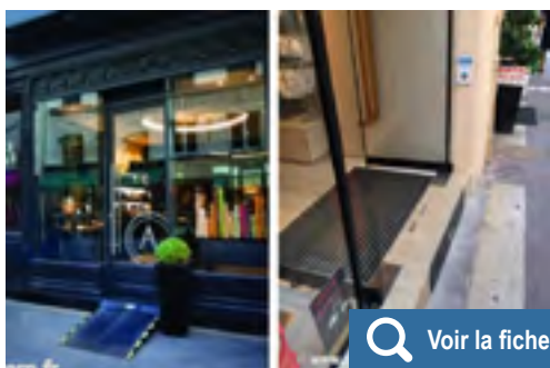
TRAIT D'UNION - RAMPE TIROIR (UNE À DEUX MARCHES) Marque : Myd'l
